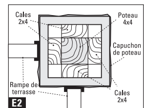
Rampe de coin
